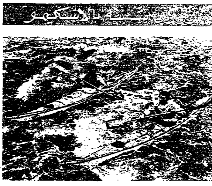
اسمه «التورنكاب» وهو مصنوع من الاليف الزجاجية والياستيك على شكل زورق لجماعة الاسكيو . ويبلغ طول الزورق الذي بنته شركة بريطانية حوالي ثلاثة امتار ونصف المتر وقد صنع خصيصا لرحلة طولها ٤.٢ كيلومتر حول «كباب هورن» في جنوبي القارة الاميركية حيث الحرارة تتعدى الى ما تحت الصفر ويصعب هبث البحار الدائم الهيجان هناك . وهذا القارب صنع بحيث يستطيع تقويم نفسه اذا انقلب وهو غير قابل للغرق
